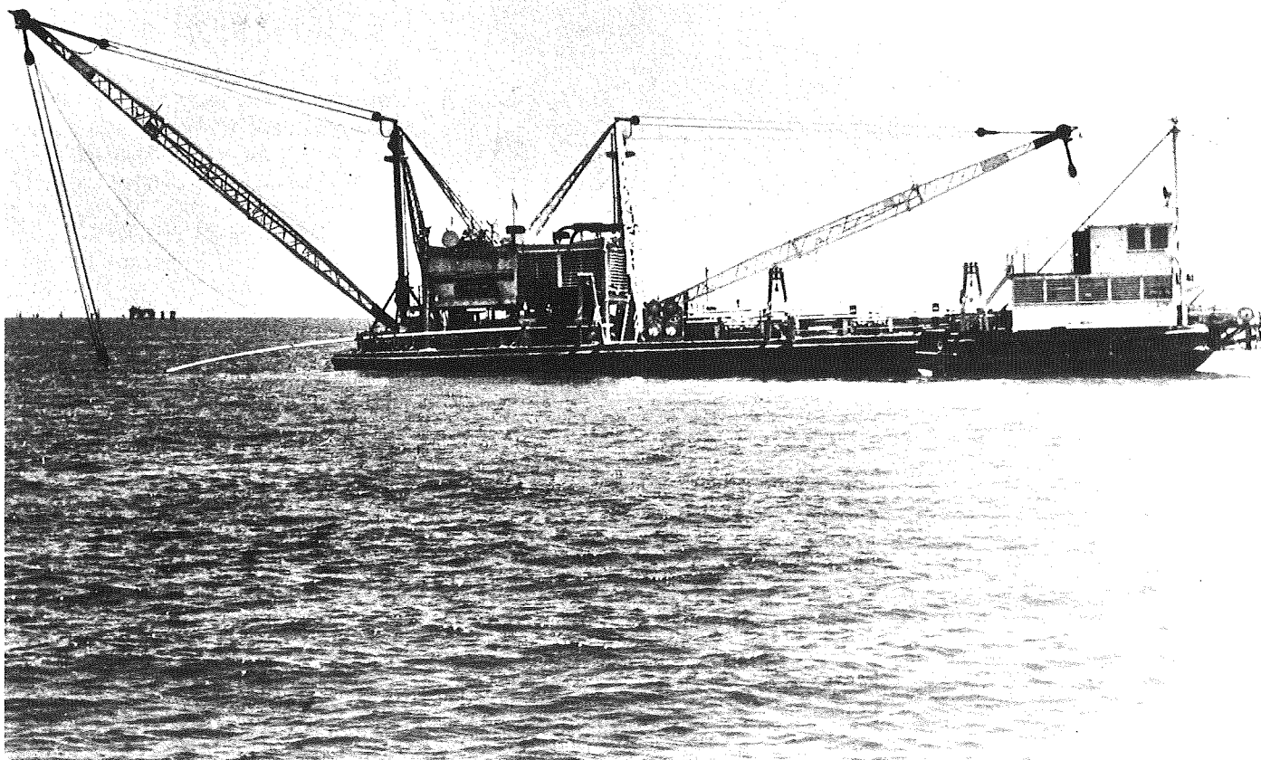
En el lago Maracaibo, los barcos extraen los tubos que conducen el petróleo desde el pozo al oleoducto.
